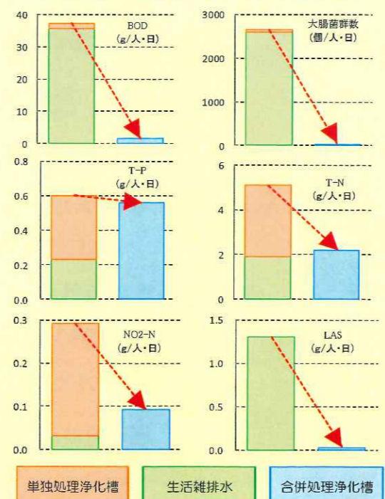
転換前後の汚濁負荷量 (1人1日あたり)
